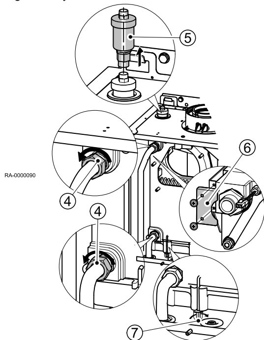
Fig.41 Fjernelse af varmeveksleren
