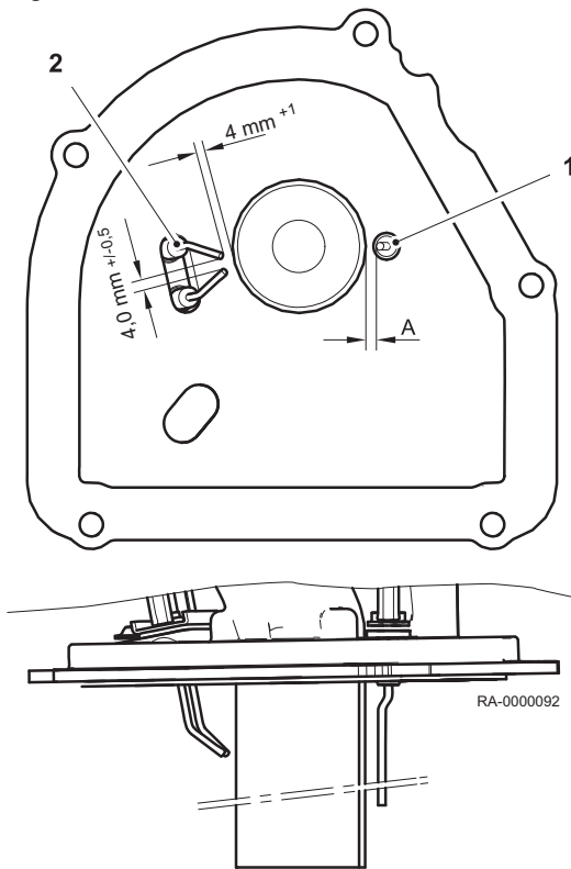
Fig.37 Elektroder
