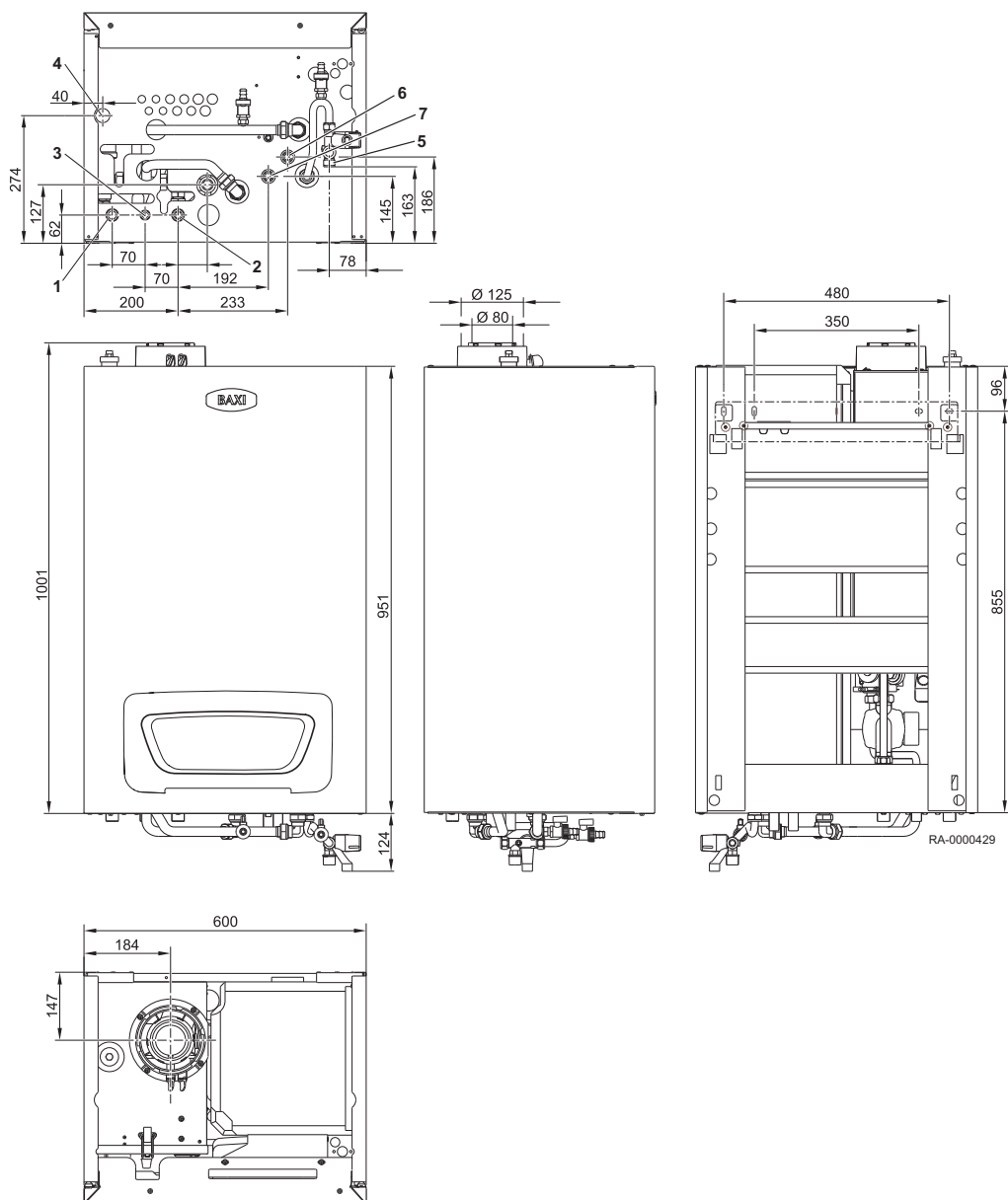
Fig.2 Mål og tilslutninger WGB-K EVO
