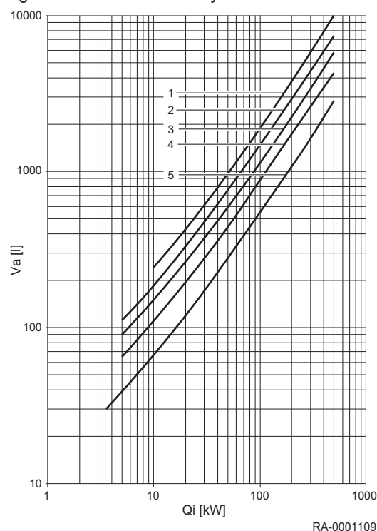
Fig.7 Fastsættelse af systemets volumen
