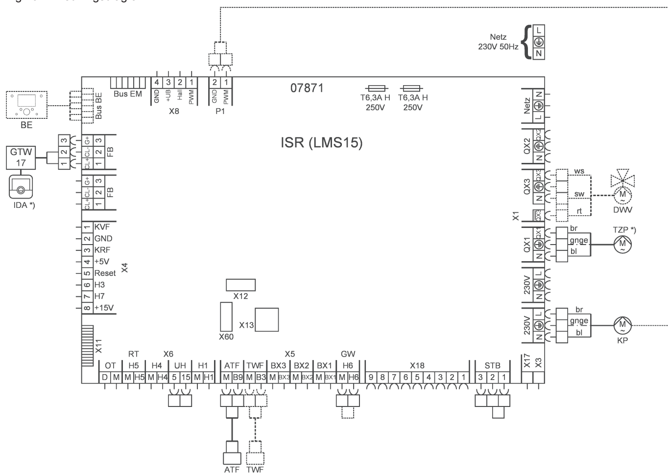
Fig.10 Ledningsdiagram
