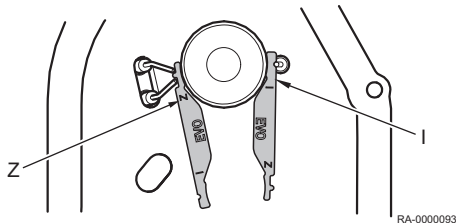
Fig.38 Kontrol af elektrodeafstande ved hjælp af afstandskabelonen
