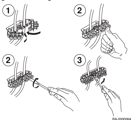
Fig.19 Aflastninger
