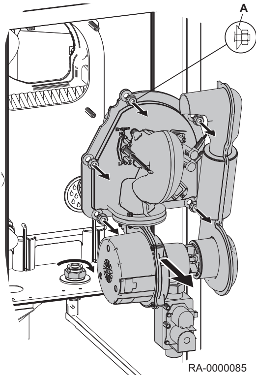
Fig.40 Fjernelse af gasbrænderen
