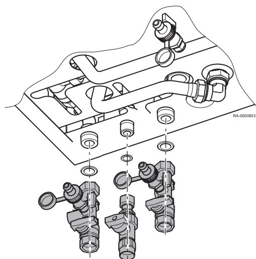
Fig.11 Installation af afbryderventiler
