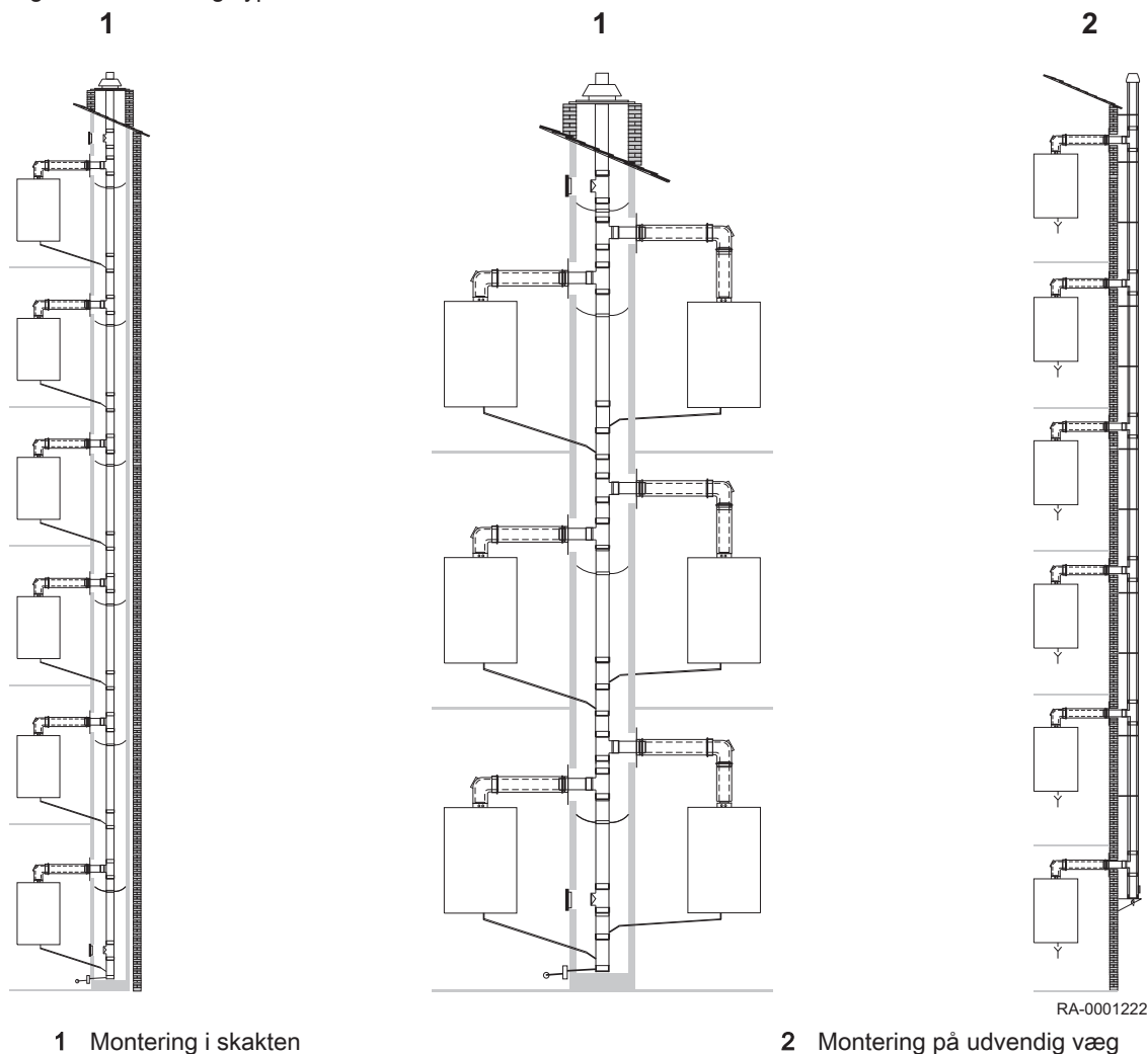
Fig.18 Monteringstyper
