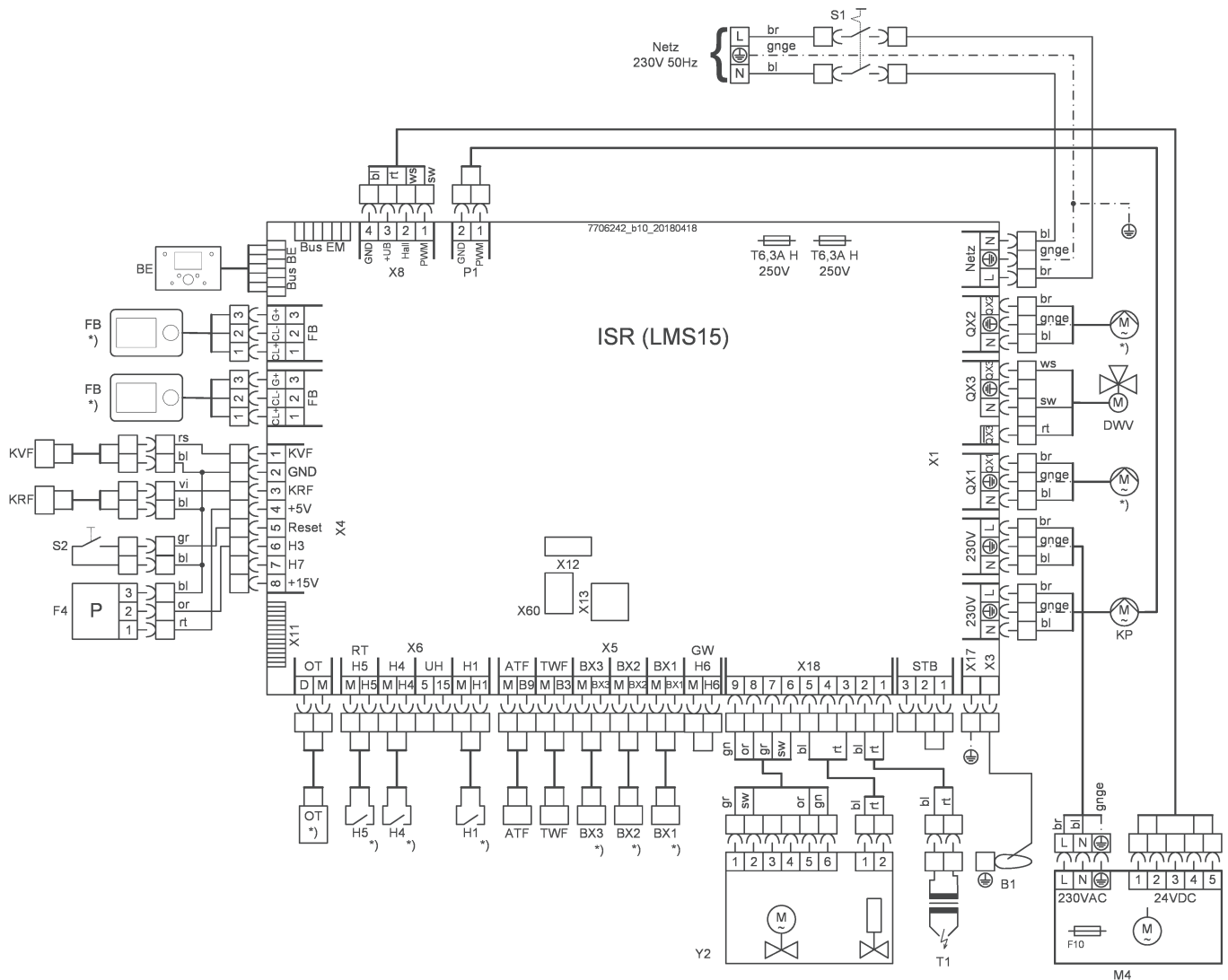
Fig.3 Ledningsdiagram WGB-K EVO
