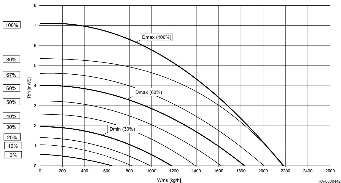
Fig.1 Samlet dynamisk højde WGB-K EVO for pumpens varmekreds
