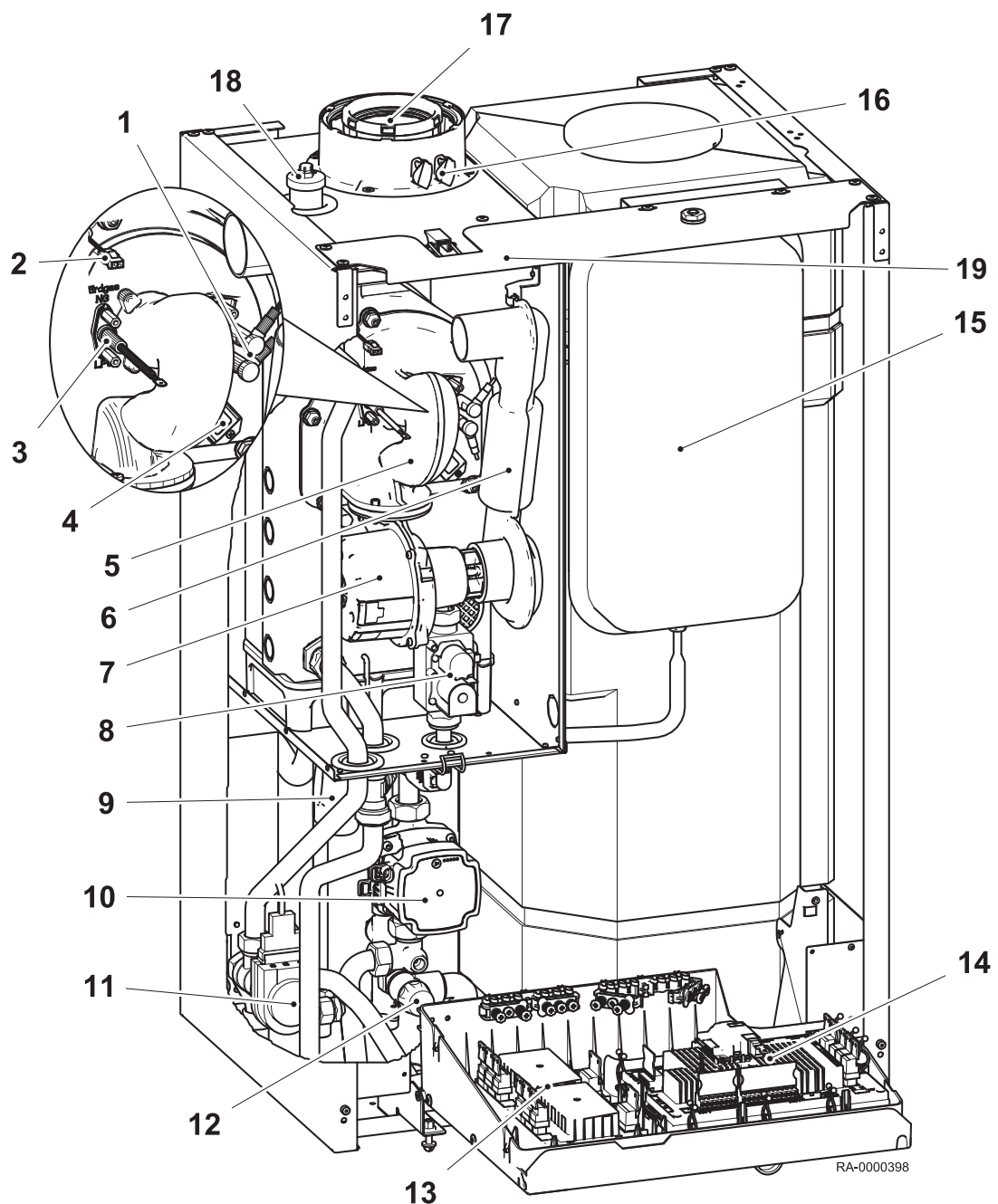
Fig.4 Kedelvisning WGB-K EVO (vises uden frontvæg og dæksel på styreenhed)
