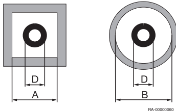
Fig.15 Skaktens minimumsmål
