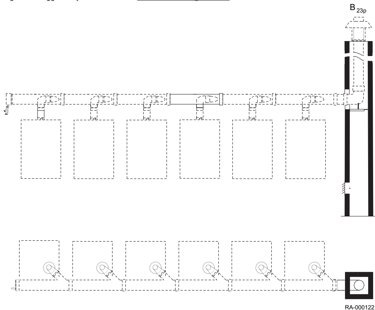
Fig.16 Røggasrørsystem til drift med åbent-forbrændingskammer
