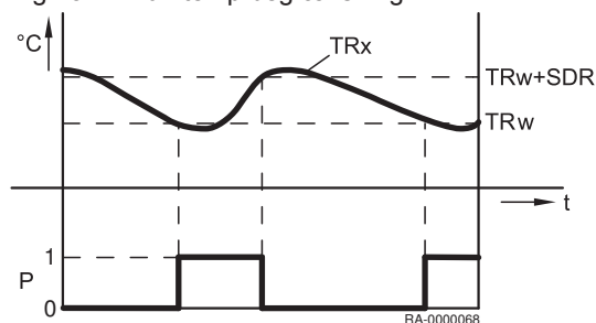
Fig.25 Rumtemp begrænsning
