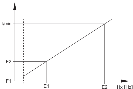
Fig.34 Eksempel på to forskellige følerkurver
