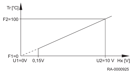
Fig.33 Spænding_værdi/Funktion_værdi
