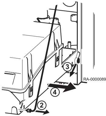
Fig.36 Afhængning af kontrolpanelet
