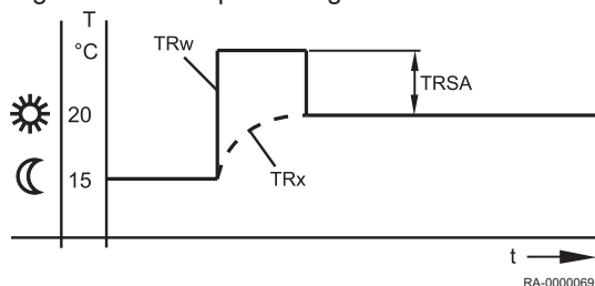
Fig.26 Boost opvarmning
