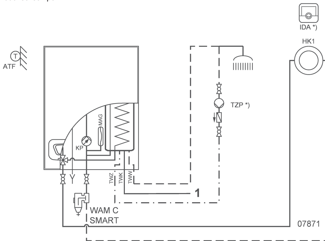
Fig.9 Applikationseksempel
