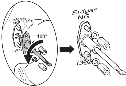
Fig.20 Skift til flaskegas
