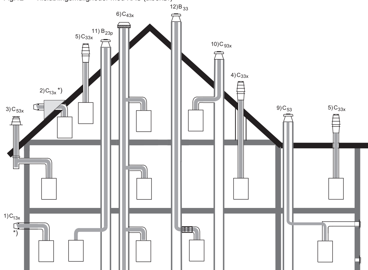
Fig.12 Tilslutningsmuligheder med KAS (tilbehør)
