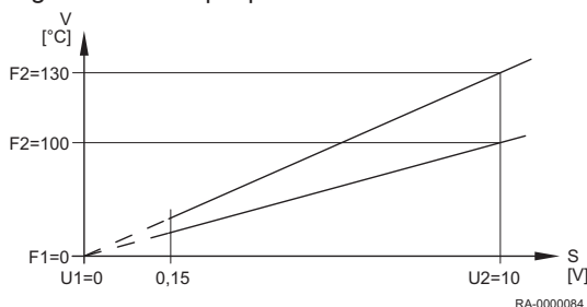
Fig.35 Eksempel på varmebehov 10 V
