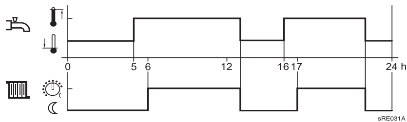
Fig.11: Frigivelse varmtvandsopvarmning afhængig af varmekredsenes tidsprogrammer (eksempel)
