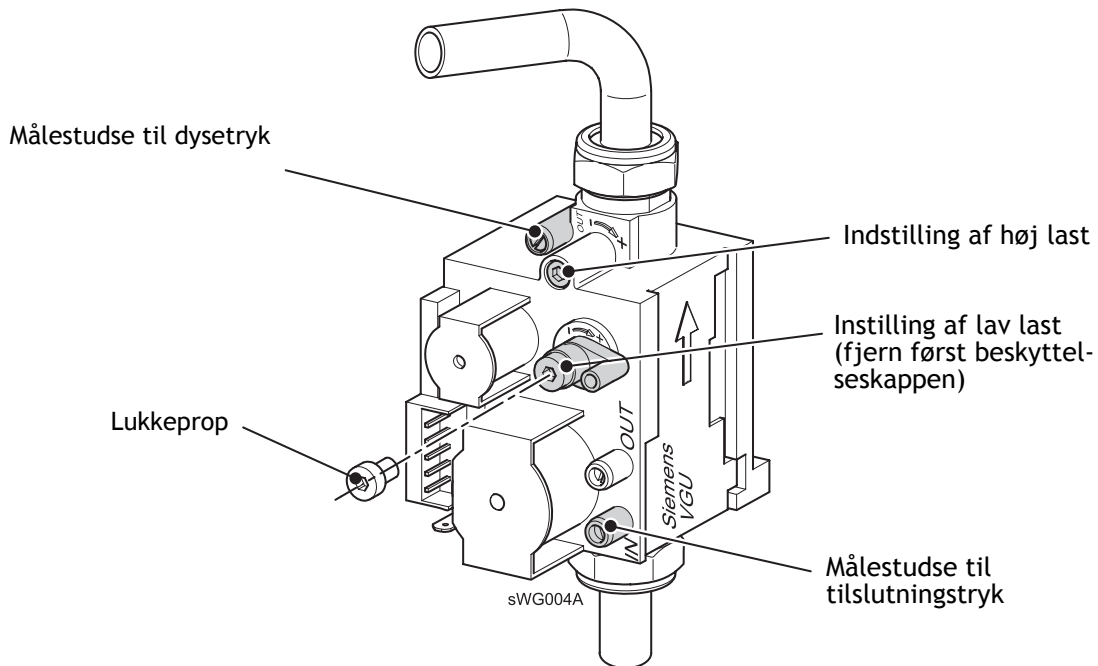
Fig.5: Gasarmatur (indstilling af dysetryk med torx T15)
