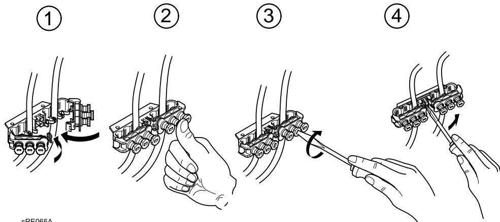
Fig.6: Trækaflastning
