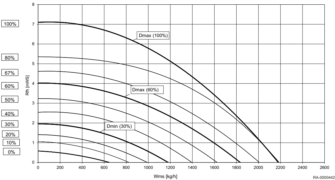
Fig.1 Samlet dynamisk højde WGB-K EVO for pumpevarmekredsløb
