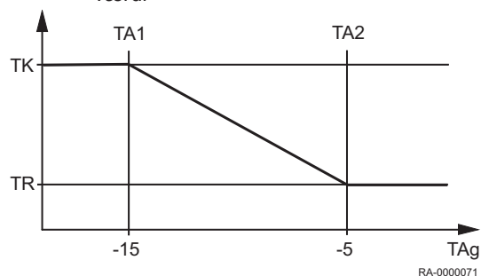
Fig.24 Forøgelse af reduceret, indstillet værdi
