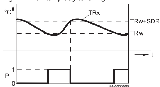
Fig.21 Rumtemp begrænsning
