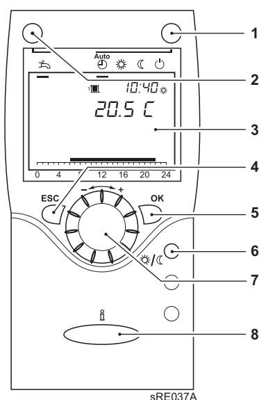
Fig.4 Driftsgrænseflade på rumenheden RGT
