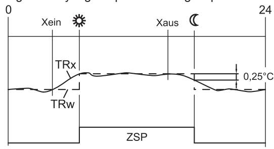
Fig.23 Styring af optimal start og stop
