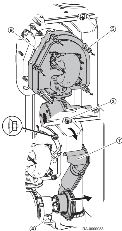
Fig.35 Fjernelse af gasbrænderen
