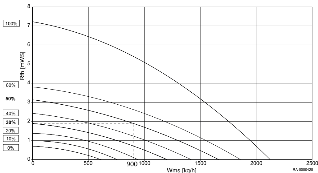
Fig.18 Eksempel på samlet dynamisk højde
