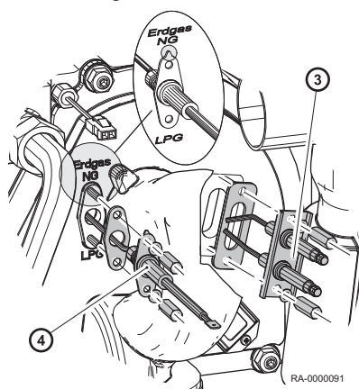
Fig.34 Fjernelse af tændings- og ioniseringselektroden
