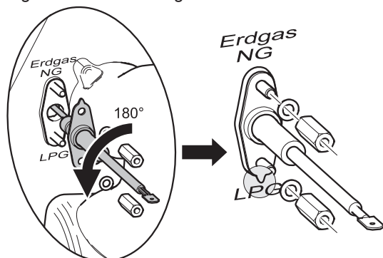
Fig.16 Skift til flaskegas
