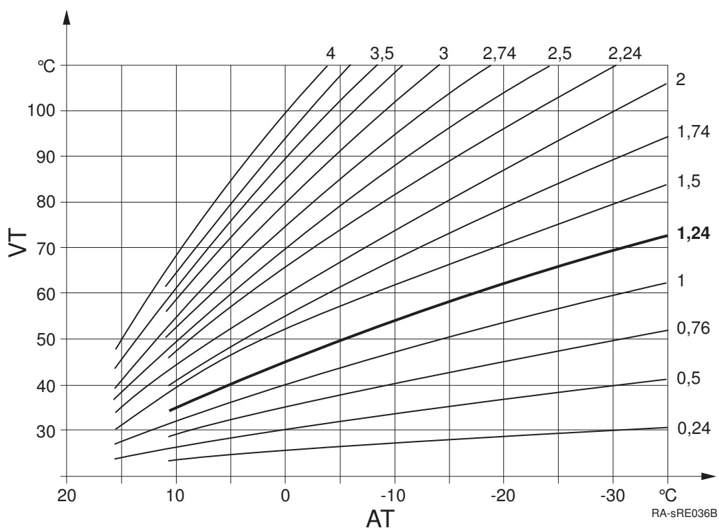
Fig.19 Varmekurvediagram
