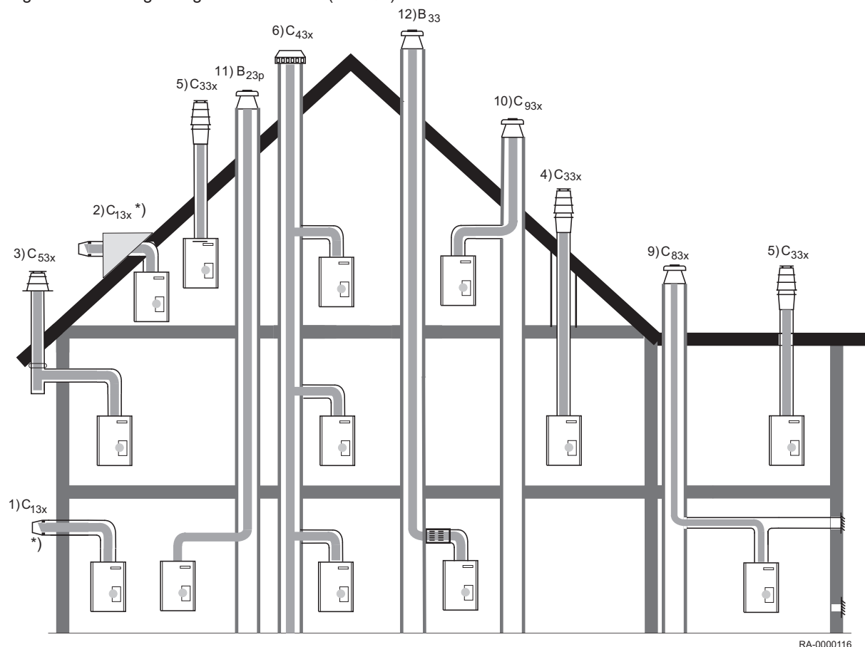
Fig.13 Tilslutningsmuligheder med KAS (tilbehør)
