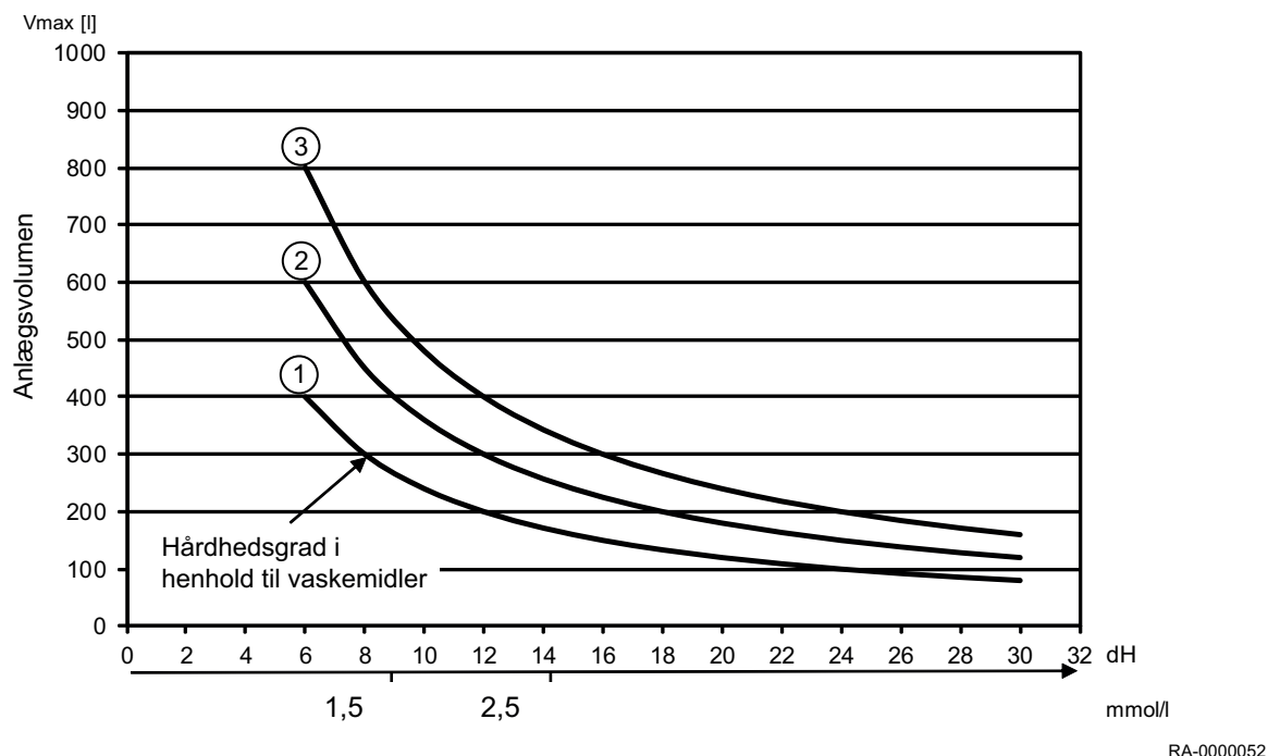
Fig.7 Diagram over vandets hårdhed
