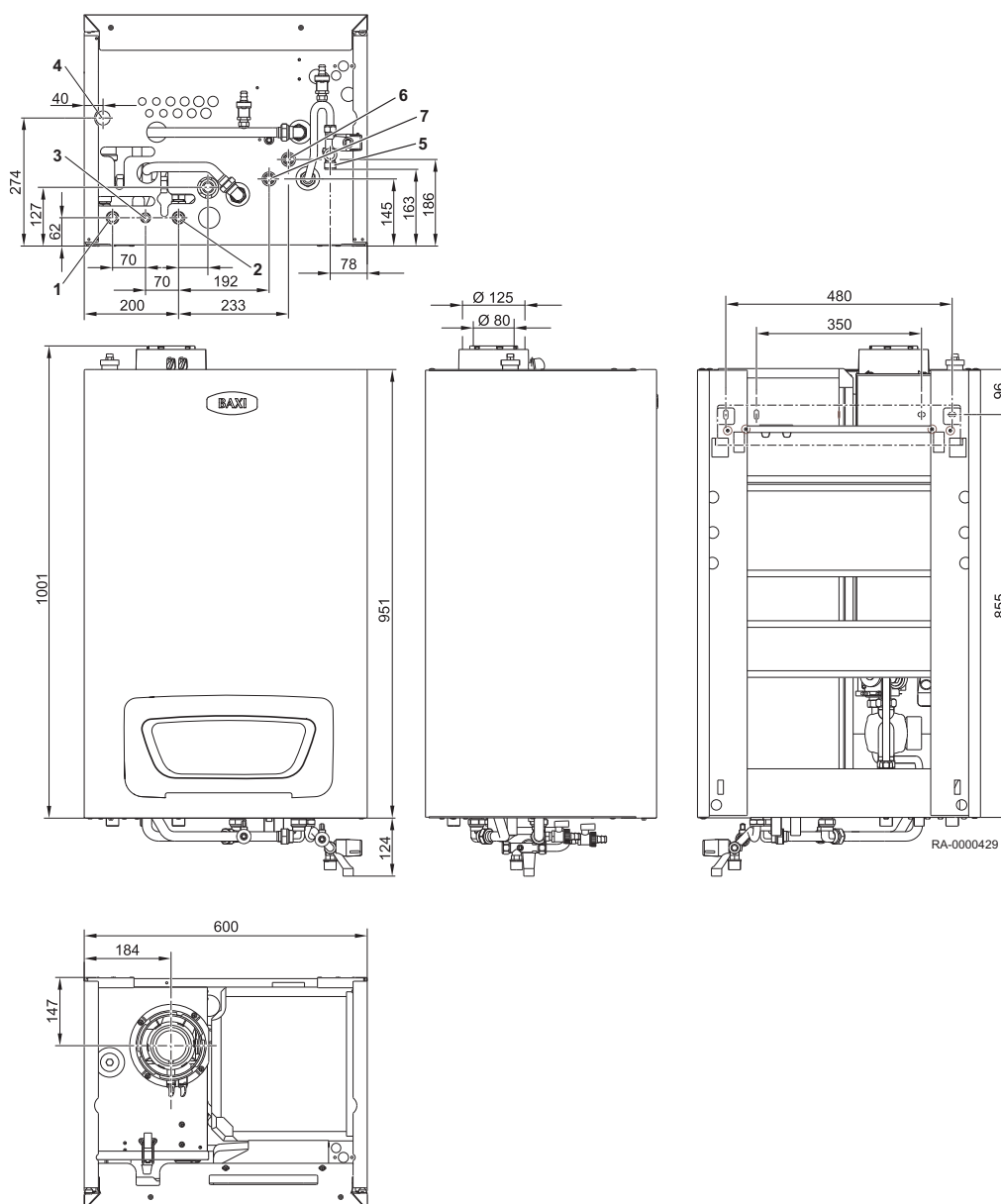
Fig.2 Dimensioner og tilslutninger WGB-K EVO
