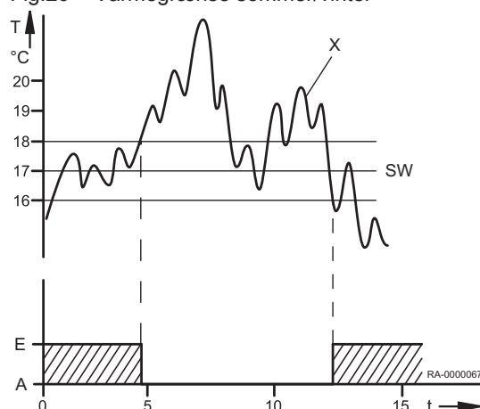
Fig.20 Varmegrænse sommer/vinter
