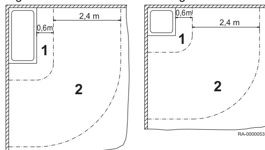
Fig.8 Frirum i badeværelser og bruserum
