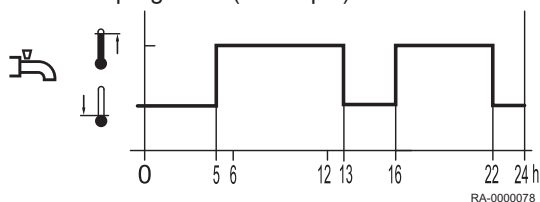
Fig.27 Frigivelse afhængigt af tidskoblingsprogram 4 (eksempel)
