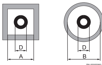
Fig.14 Skaktens minimumsmål:
