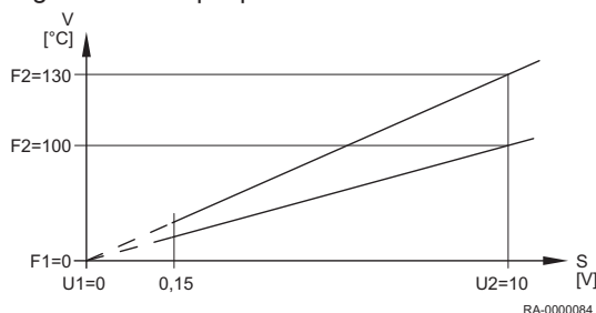
Fig.31 Eksempel på varmebehov 10 V
