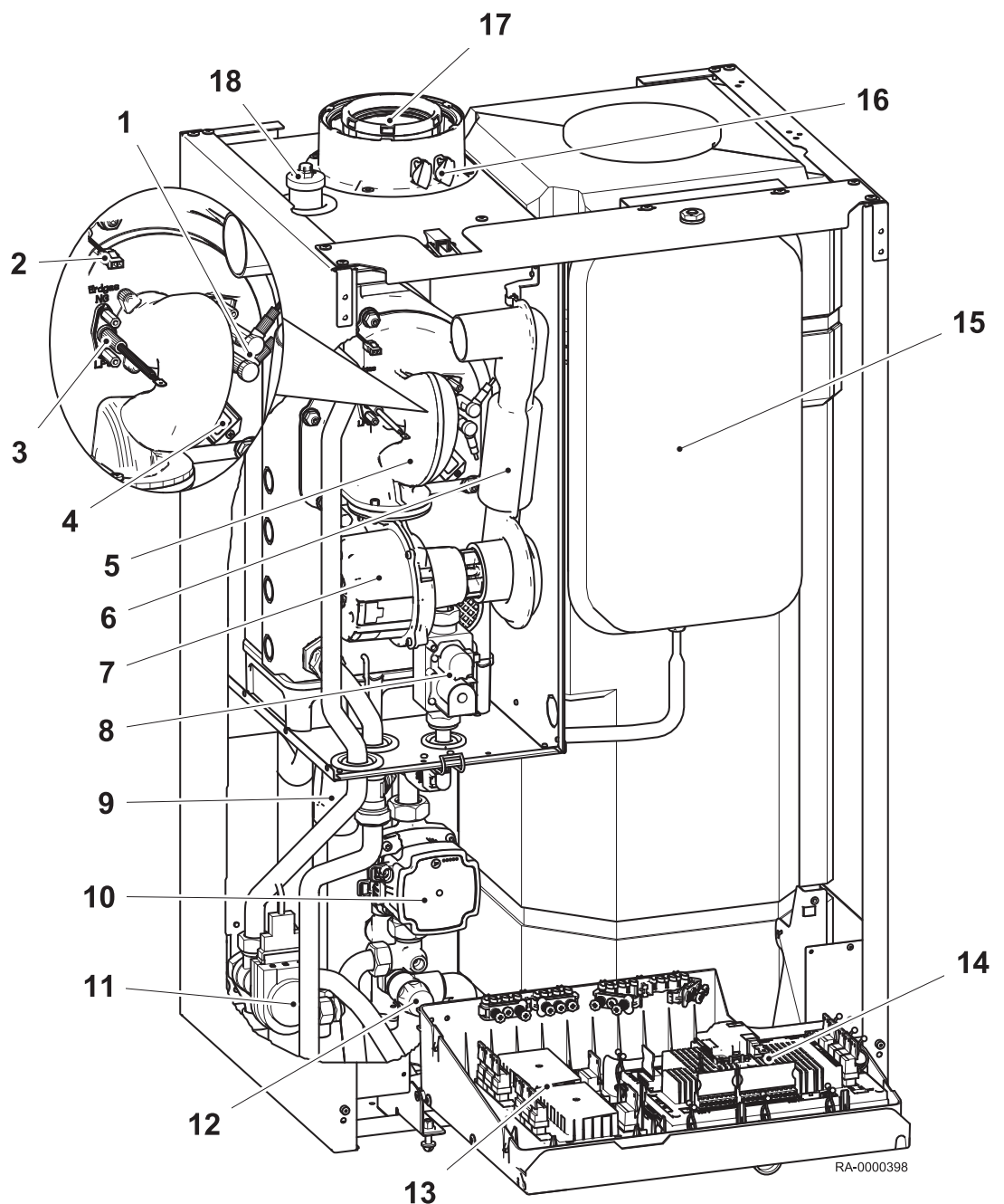
Fig.3 Kedelvisning WGB-K EVO (vises uden frontvæg og regulatordæksel)
