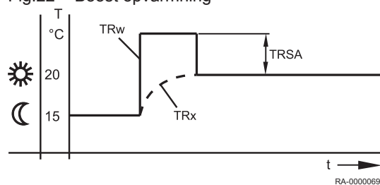
Fig.22 Boost opvarmning
