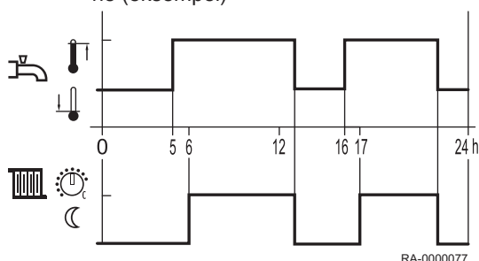
Fig.27 Frigivelse afhængigt af tidskoblingsprogram 4 (eksempel)
