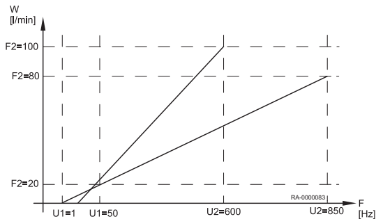
Fig.30 Eksempel på to forskellige følerkurver
