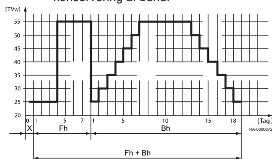
Fig.25 Temperaturprofil på funktionen til konservering af bund.
