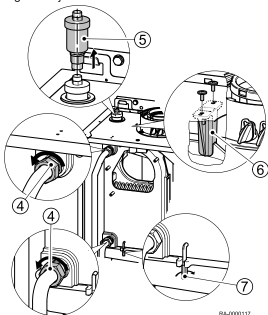
Fig.36 Fjernelse af varmeveksleren
