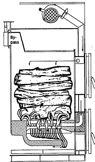
Fig. 1.3.13 #4 Korrekt indstilling Flammens farve er gul og let blålig
