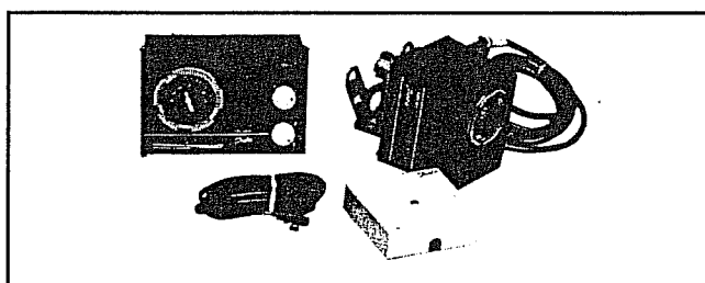
Fig. 2.2 Danfoss ECL
