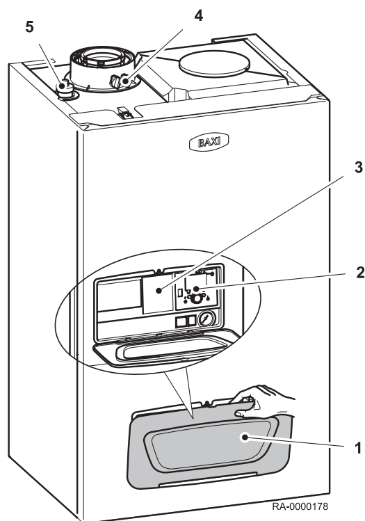
Fig.1 Oversigtsskema WGB-K EVO
