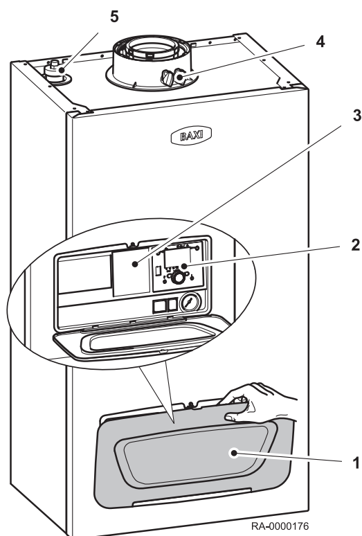
Fig.1 Oversigtsskema WGB EVO
