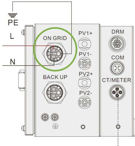
Ill. 4.1 - Tilslutning af AC.
