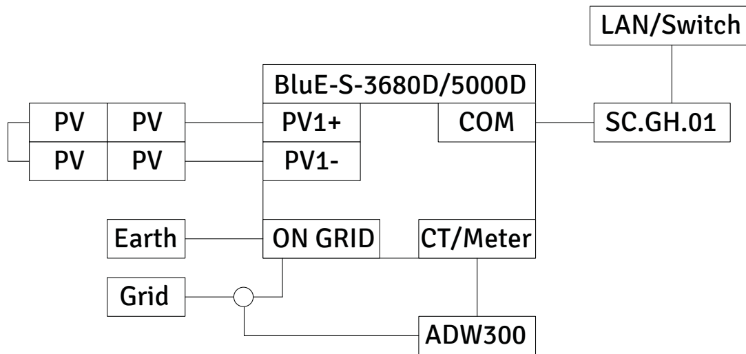
Ill. 3.1 - Principtegning med BluE-S-3680D hybridinverter.
