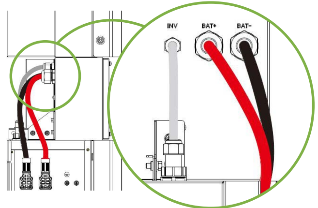
Ill. 4.3 - Tilslutning af batteri.
